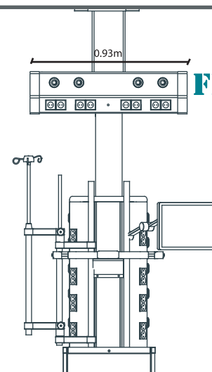
SLIDING PENDANT
